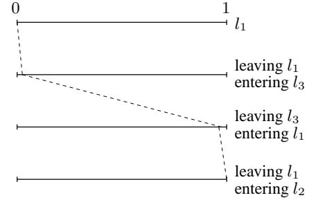
Fig. 9. The run \rho_2(\varepsilon, 1 - 2 \cdot \varepsilon, \varepsilon)
